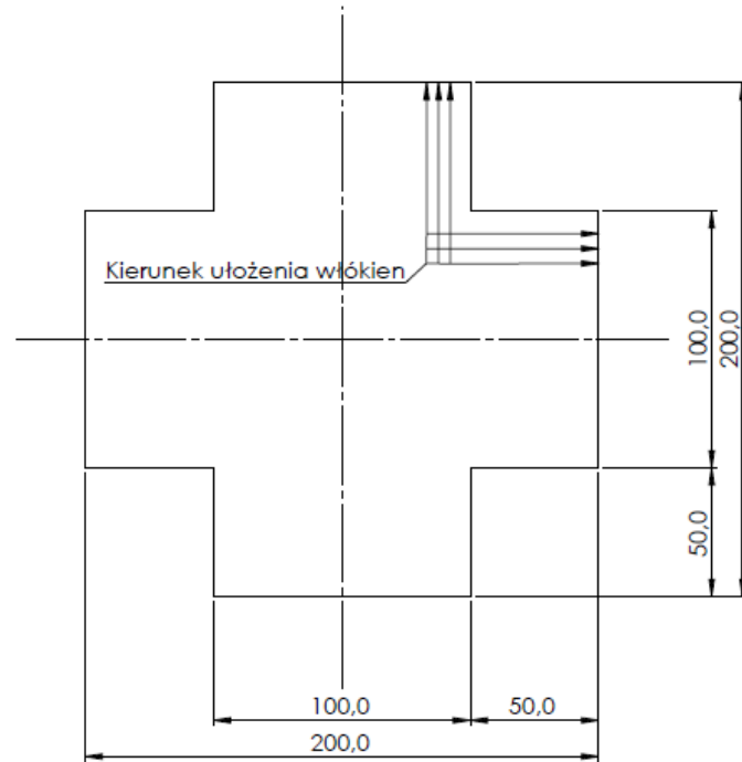
Rys. 4.9. Nominalny kształt i wymiary próbki pojedynczej warstwy materiału włóknistego
