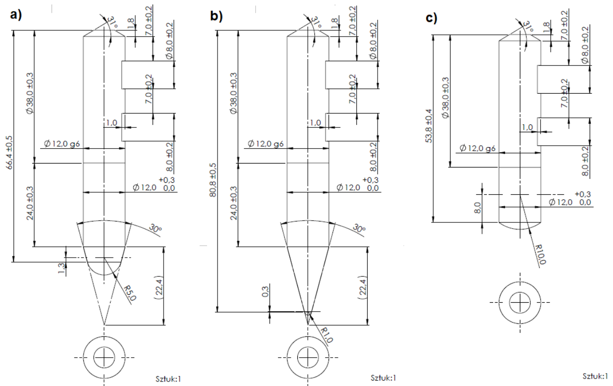
Rys. 4.10. Narzędzia do punktowego obciążenia tkaniny (penetratorów) o promieniu:
