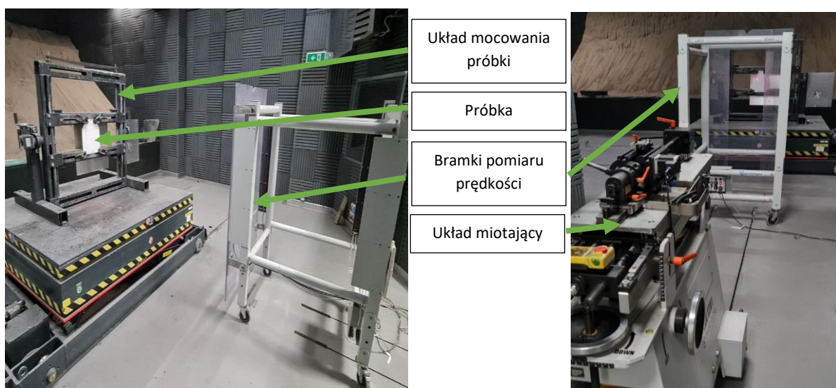
Rys. 5.5. Stanowisko badawcze do ostrzały odłamkiem standardowym FSP
