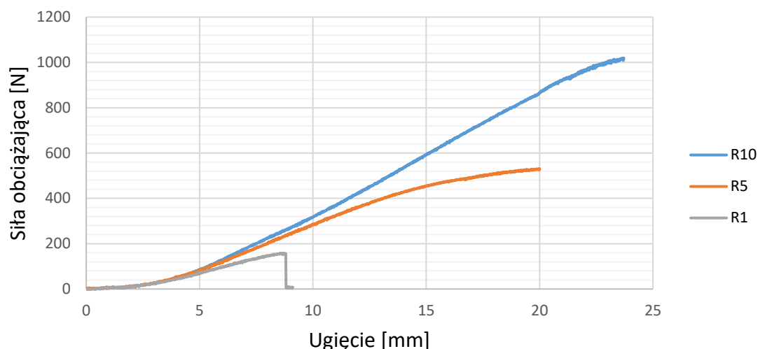
Rys. 5.2. Wpływ różnych narzędzi do badania poprzez obciążenie punktowe próbki Teijin UD
