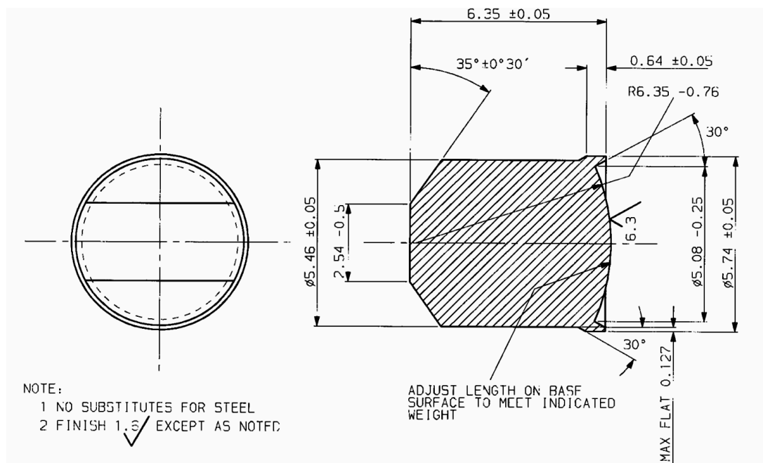
Rys. 1.1. Odłamek kalibru .22 – 1.1g (do ostrzału bez sabotu)[16]
