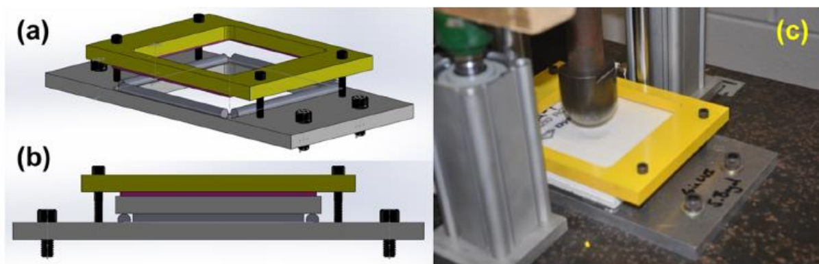
Rys. 1.5. Układ do badań uderowych o niskiej prędkości z swobodnie podpartymi warunkami brzegowymi do płaskich paneli UHMWPE. Schemat mocowania (a) bez próbki, (b) widok z boku z próbką i (c) na miejscu na wieży do obciążników Dyantup z zamocowaną próbką i penetratorem kulistym o średnicy 5,1 cm [27]
