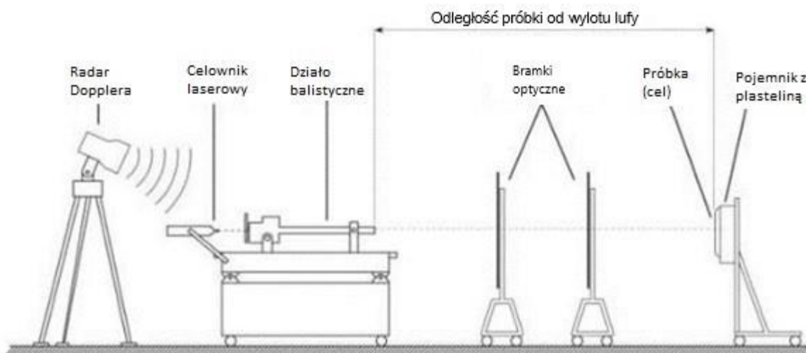
Rys. 4.14. Schemat stanowiska eksperymentalnego stosowanego do badań balistycznych na odporność balistyczną V_{50}
